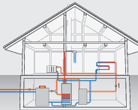
Schema Sole-Wärmepumpe
